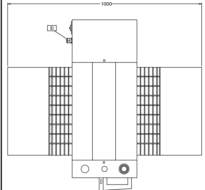
Boven aanzicht
